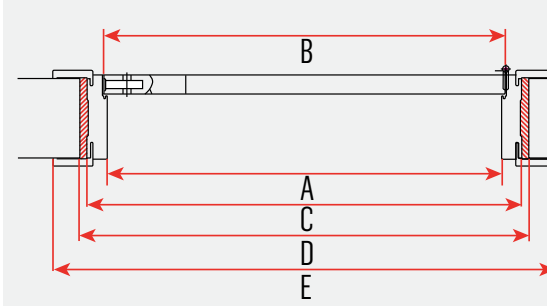
RESİM 1: KAPI GENEL KESİT
