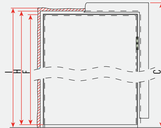
RESİM 2: KAPI YÜKSEKLİKLERİ
