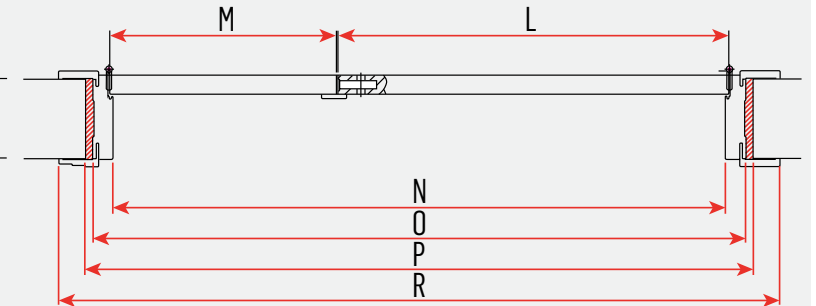
RESİM 3: SALON KAPISI GENEL KESİT
