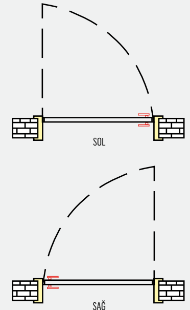
RESİM 3: SALON KAPISI GENEL KESİT
